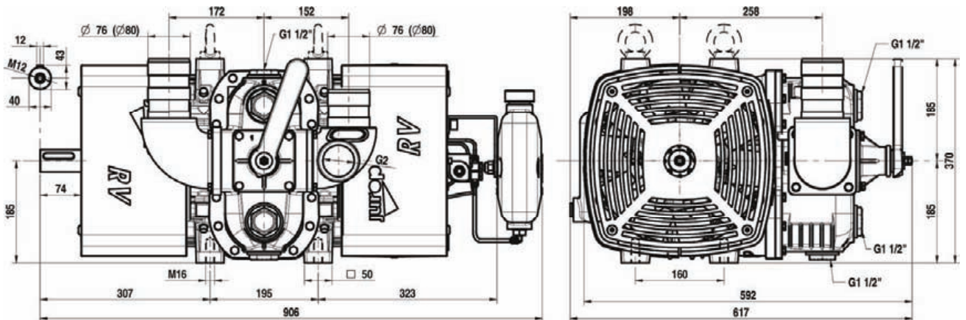
Abmessungen JUROP Vakuumpressor RVC 360
