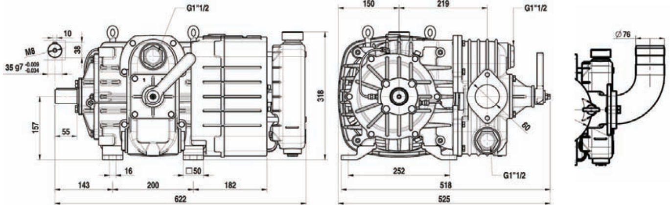
Abmessungen JUROP Vakuumpressor RVC 210
